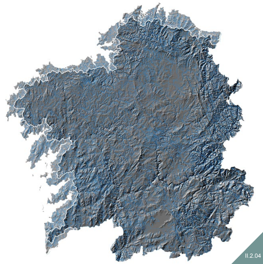
II.2.04 Cartografía da rede fluvial
