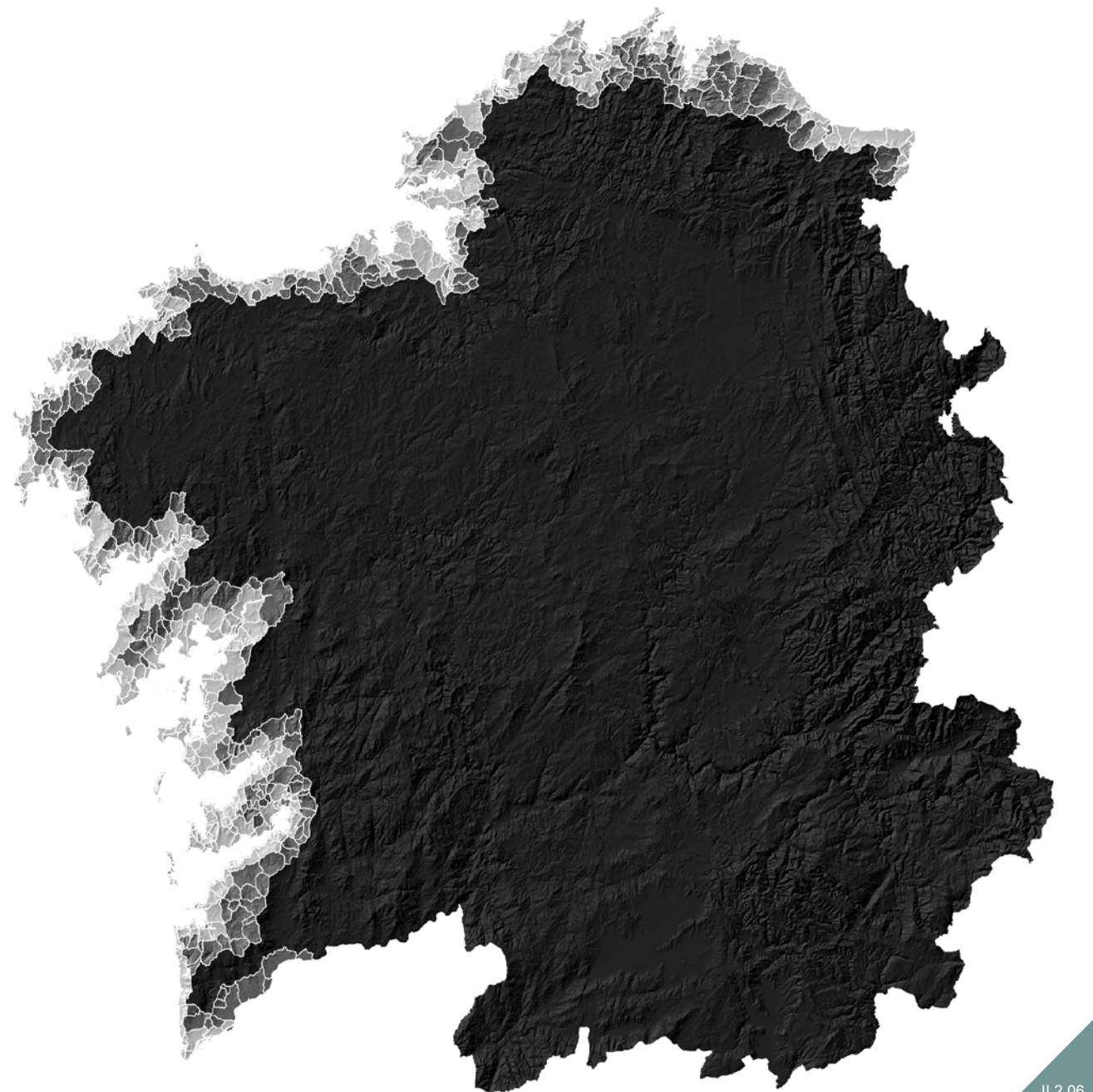
Modelo dixital do terreo distinguindo as unidades litorais e prelitorais
