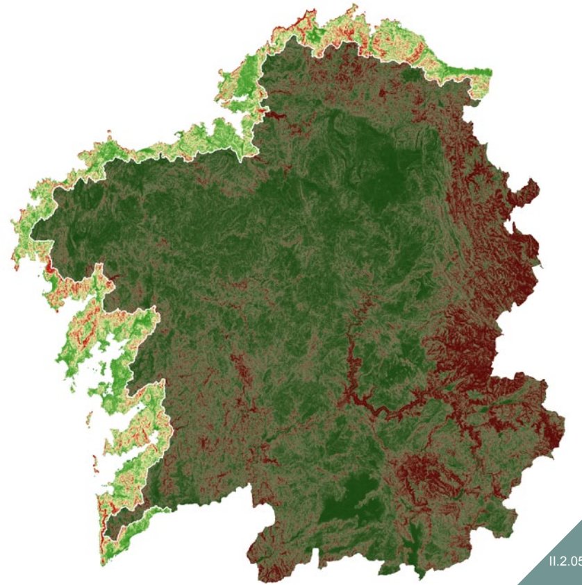
II.2.05 Mapa de pendentes
