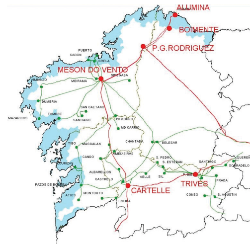
Rede de transporte.
