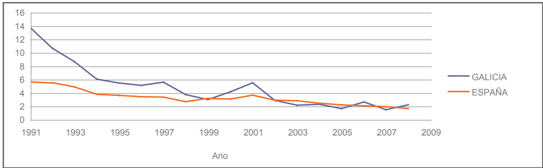
Comparación TIEPI Galicia-España.
