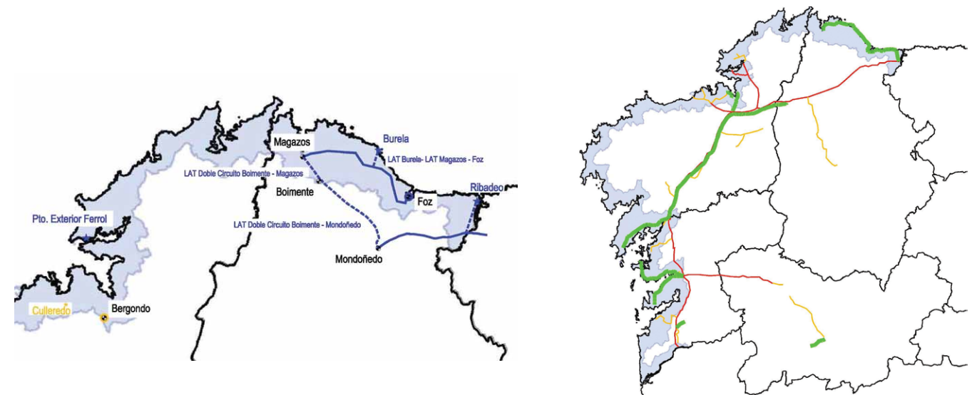
Previsións 132 kV (azul) e 66 kV (amarelo) zona norte.
