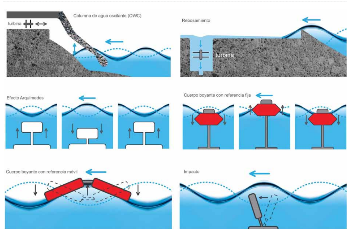
Clasificación dos sistemas de aproveitamento undimotriz. FONTE: European Wave Energy Atlas.
