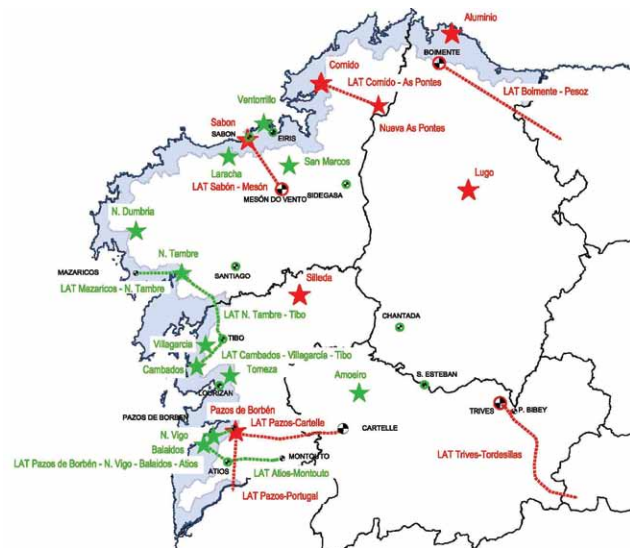
Novas Infraestruturas de transporte.
