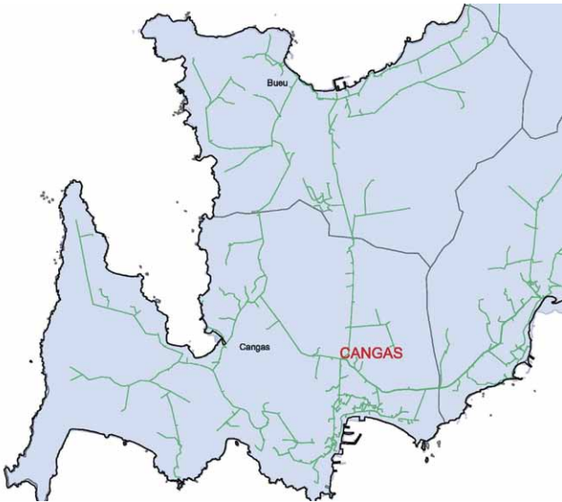
Mallado de 20 kV na zona do Morrazo.
