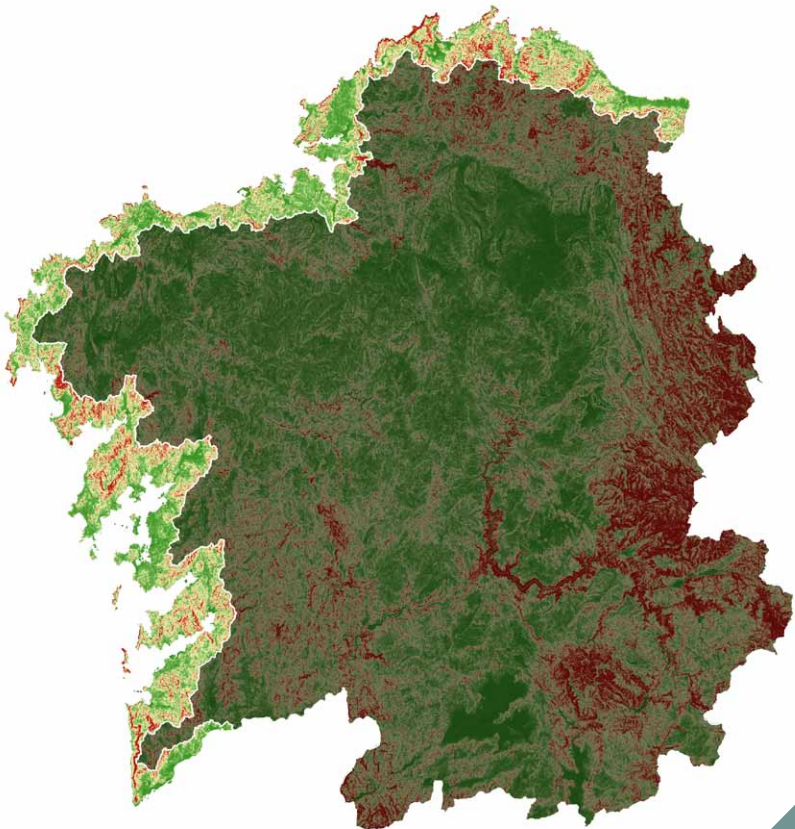
Mapa de pendentes
