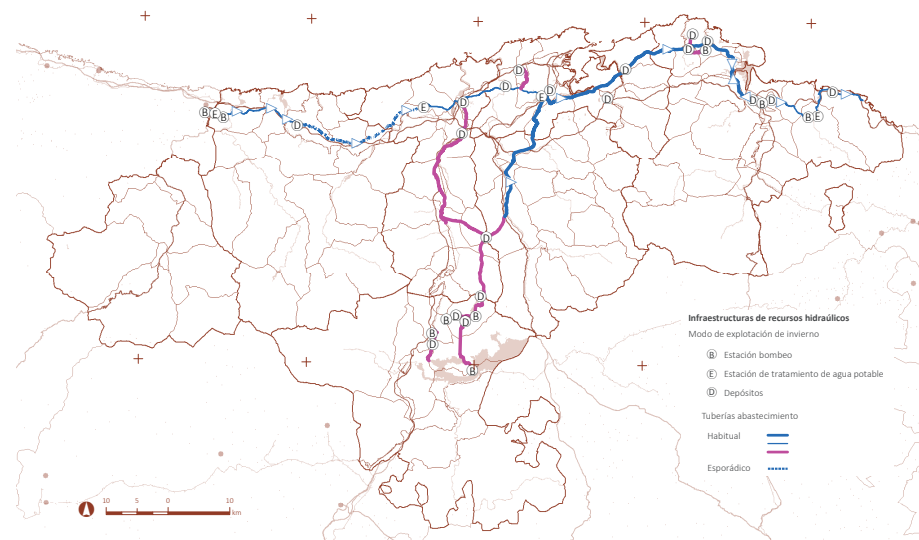
Figura 43. Autovía del agua y Bitrasvase Plan General de Abastecimiento y Saneamiento de Cantabria (PGAS), 2015.
