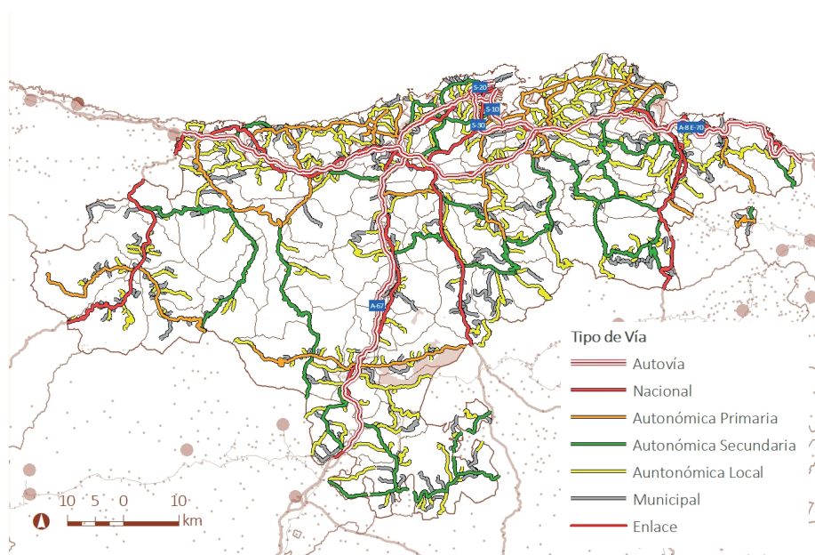
Figura 34. Red viaria Dirección General de Obras Públicas.
