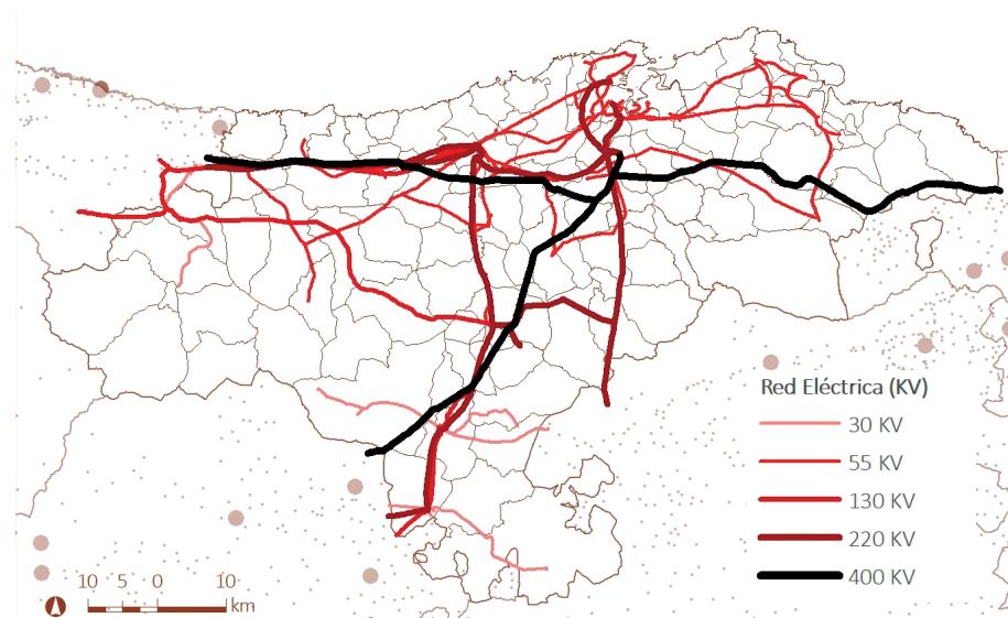
Figura 4.1. Red eléctrica Elaboración a partir de Gobierno Regional.
