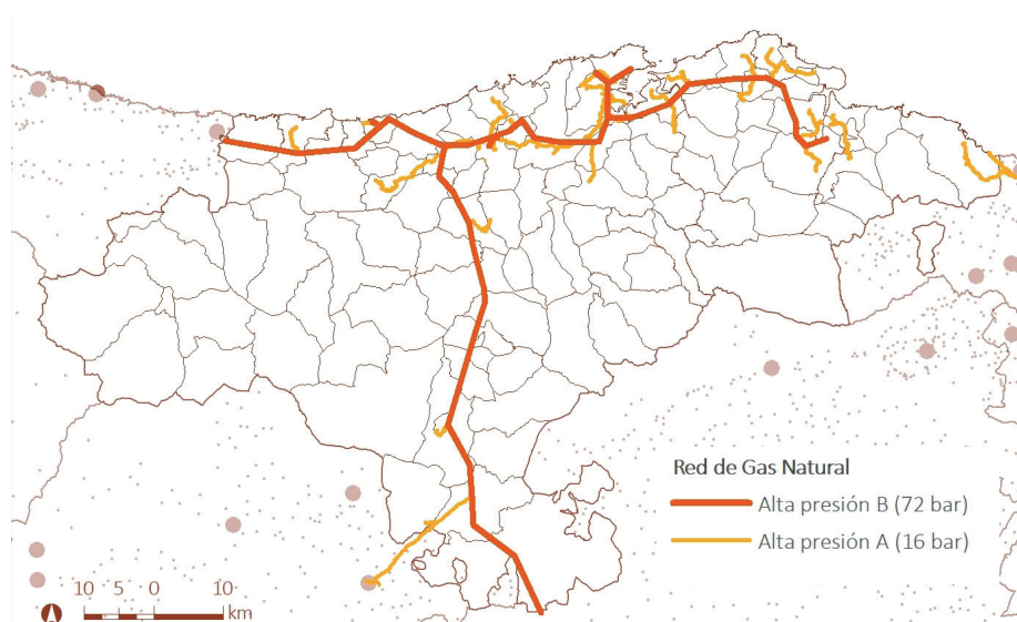
Figura 4.2. Red de gas Elaboración a partir de HC Energía, 2012.
